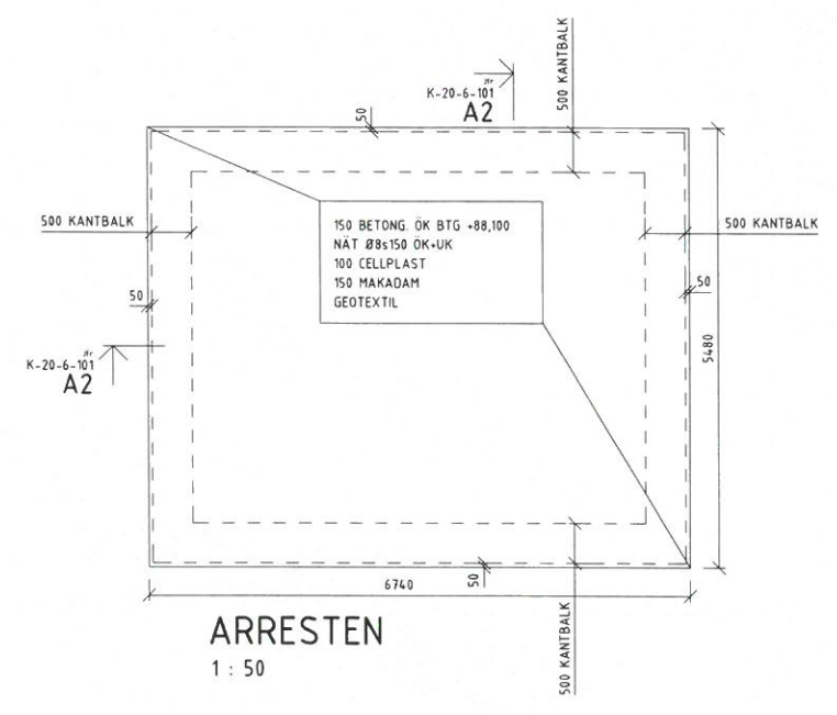
TINGSHUSET 1 : 50
