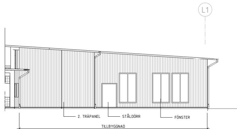
FASAD MOT ÖSTER
