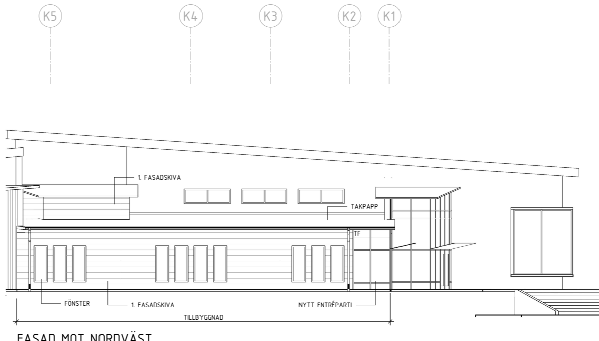
FASAD MOT NORDVÄST
