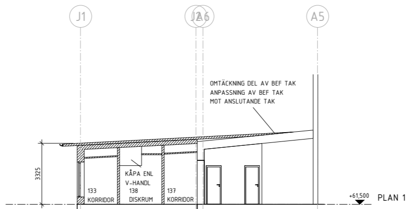
SEKTION C-C
