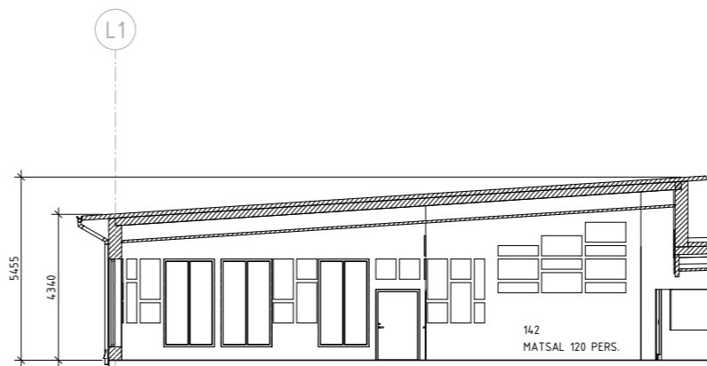
SEKTION D-D
