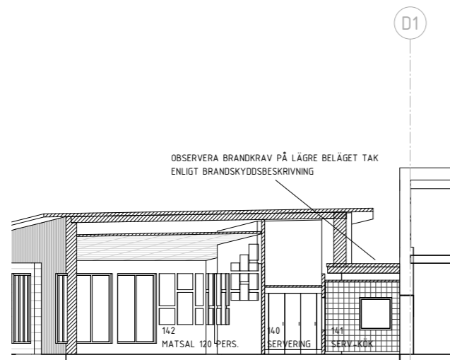
SEKTION B-B
