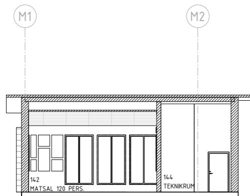
SEKTION A-A
